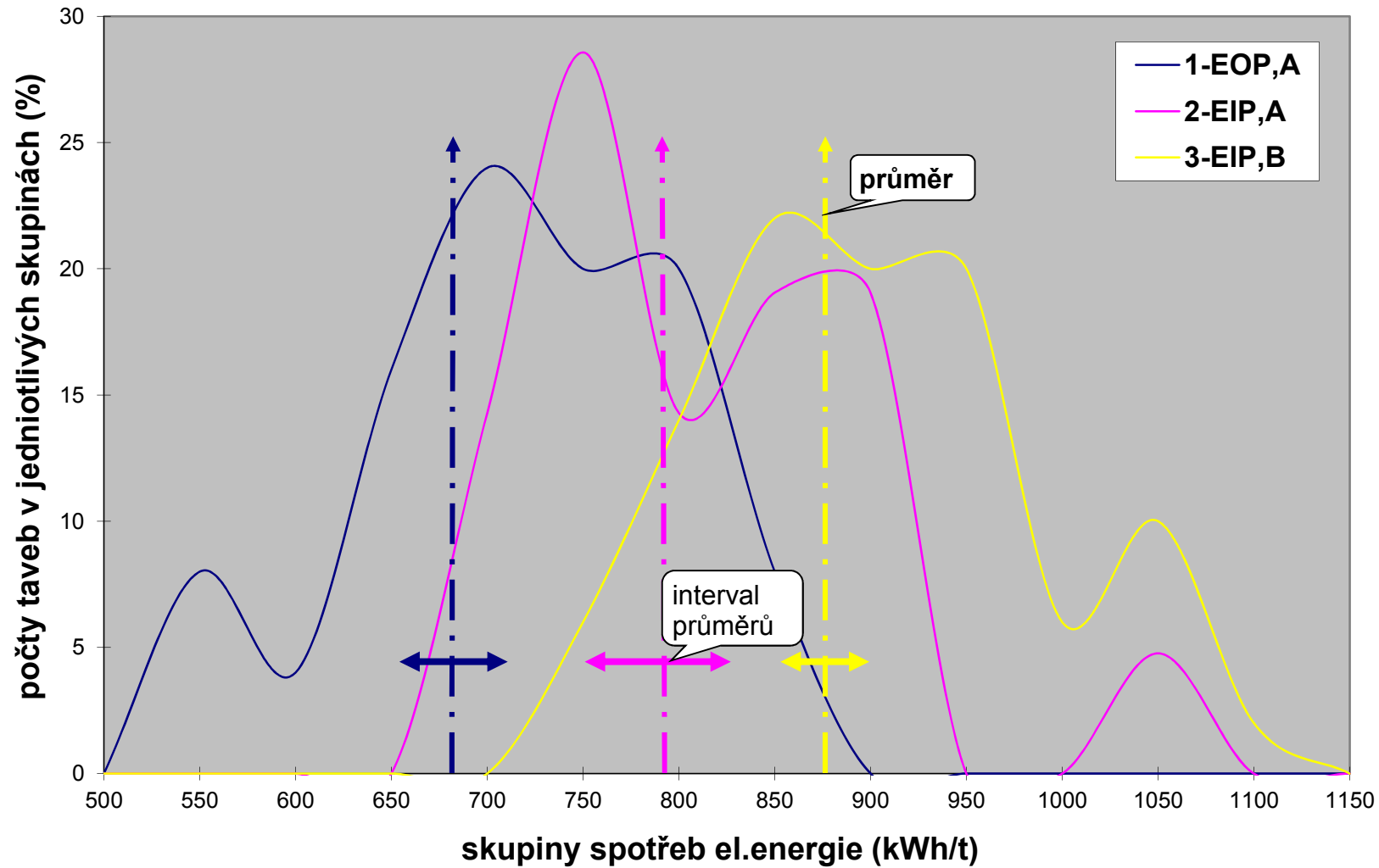
Obr. 4a: Relativní četnosti spotřeby el.energie (kWh/t)
