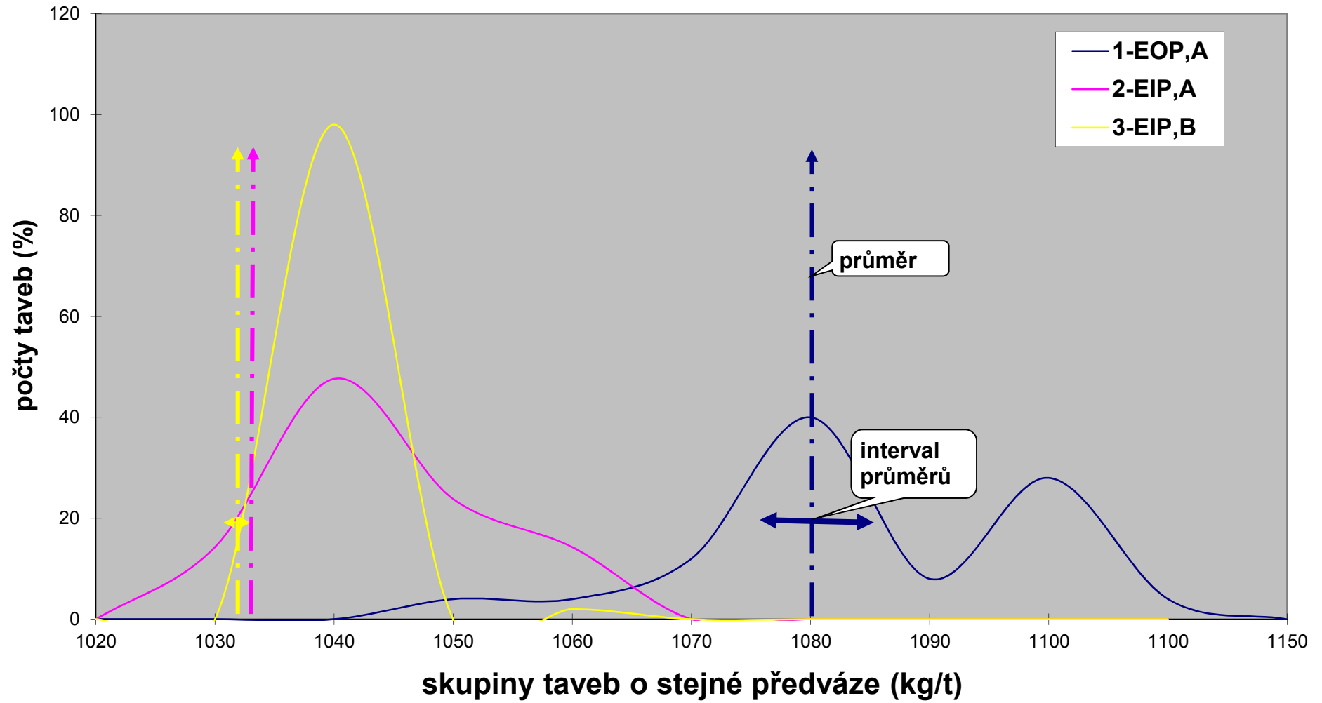
Obr.5a: Relativní četnosti předváhy u výrobních způsobů "OCEL"
