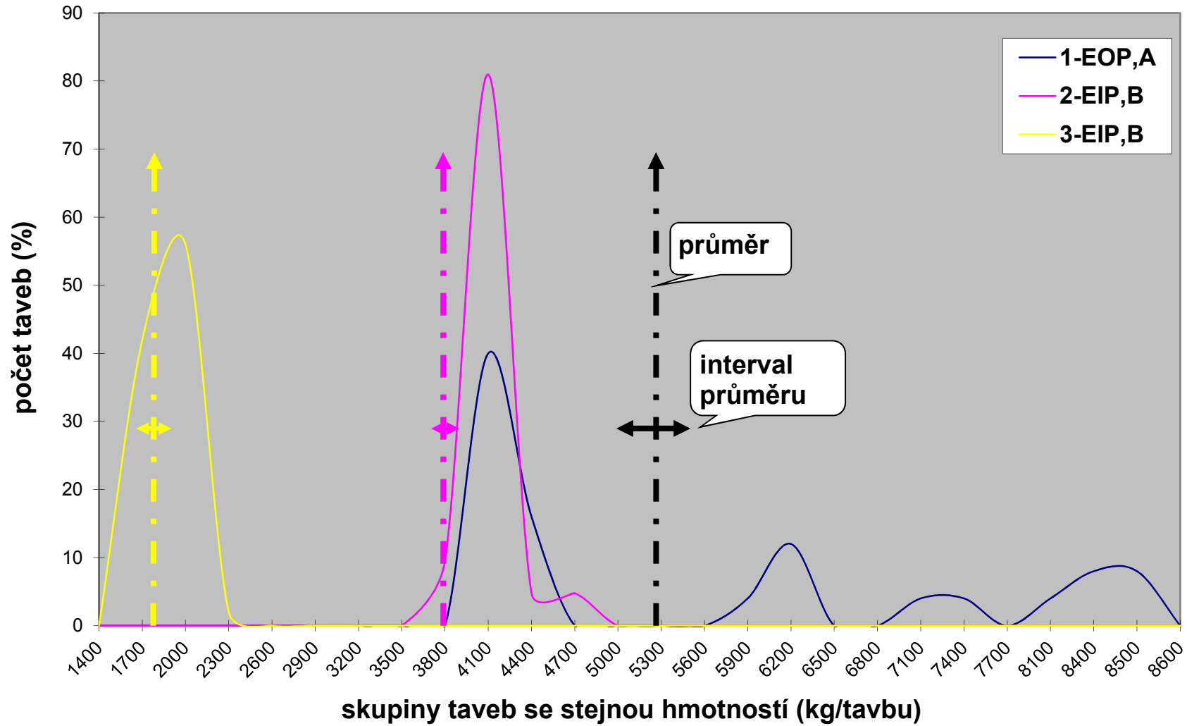
Obr. 7a: Relativní četnosti hmotnosti odlitého kovu u výrobních způsobů "OCEL"
