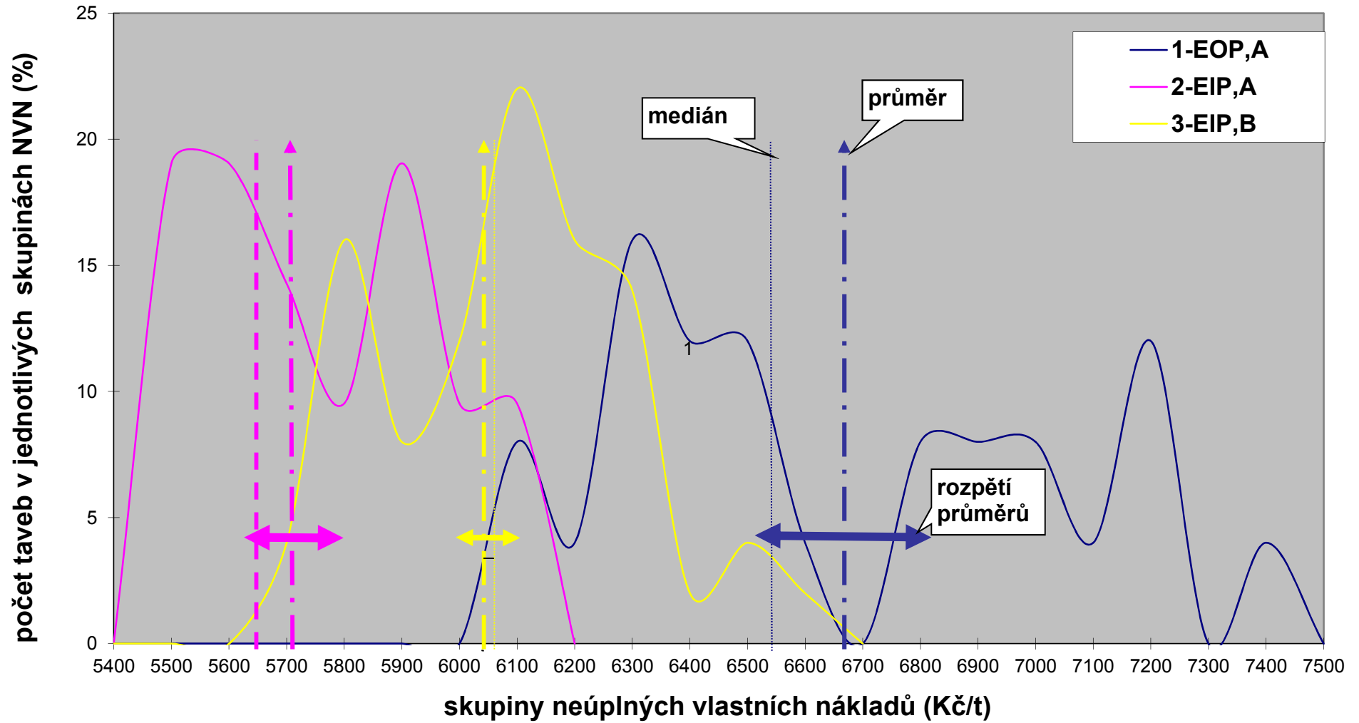
Obr.1a: Relativní četnosti NVN výrobních způsobů "OCEL"
