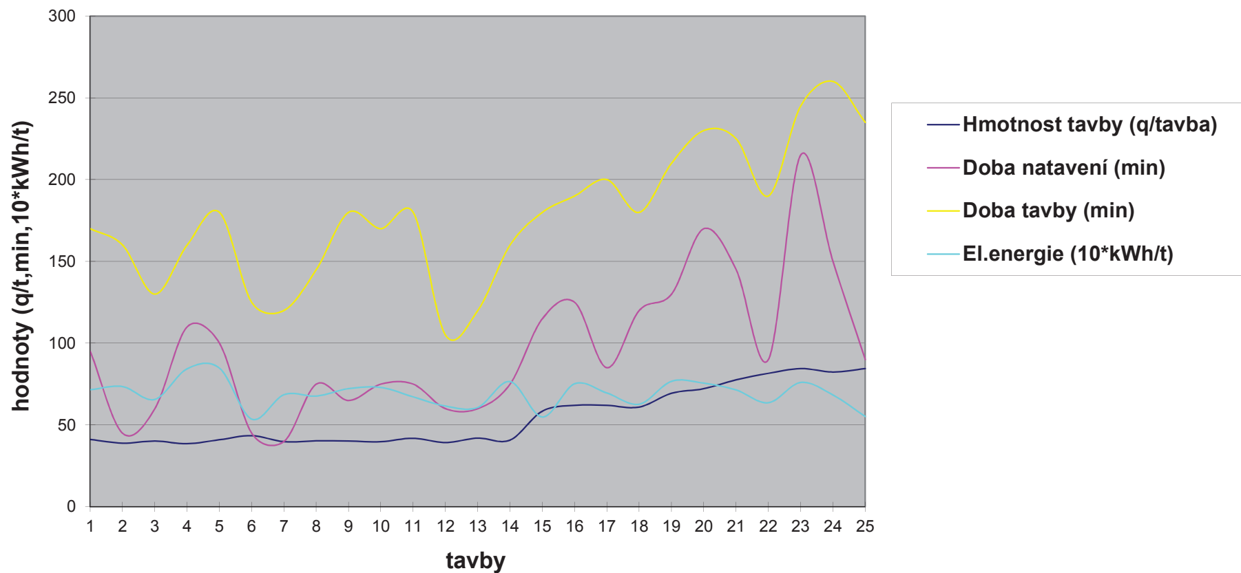
Obr. 8a: Závislost doby natavení ,tavby a spotřeby el.energie na hmotnosti tavby u VZ 1
