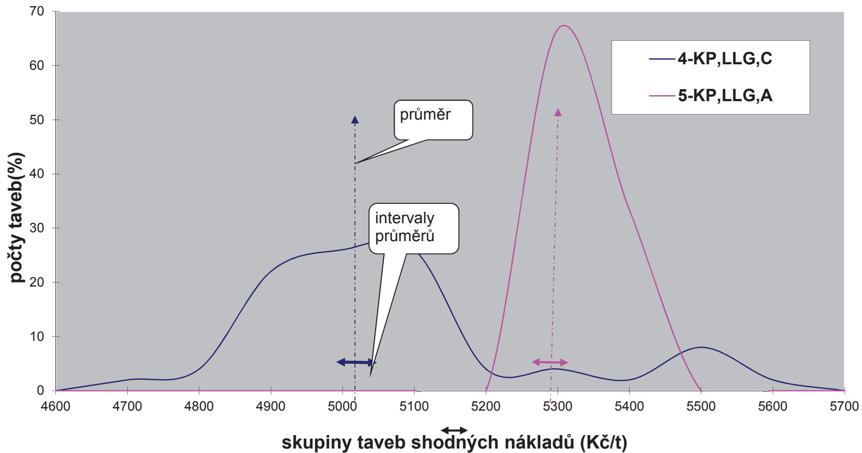
Obr. 2b: Relativní četnosti nákladů na vsázku a přísady u výrobních způsobů "LLG"
