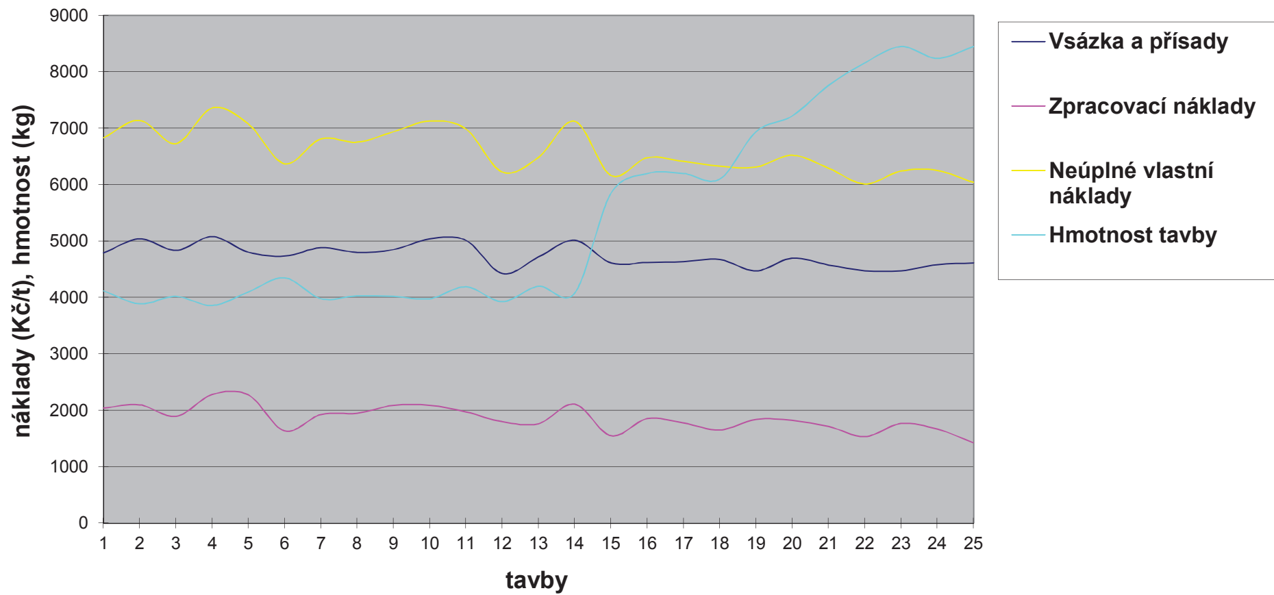
Obr.9a: Závislost nákladů na hmotnosti tavby u VZ 1
