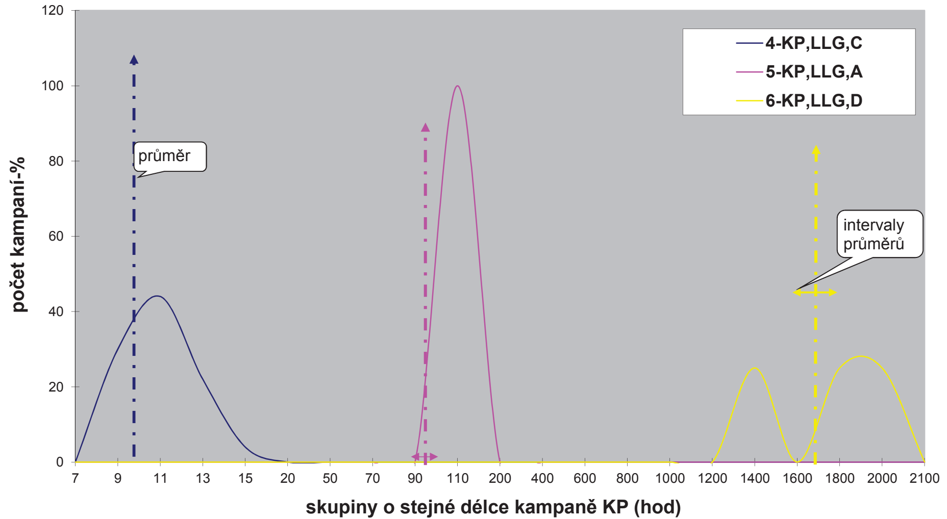
Obr.6b: Relativní četnosti délky kampaně u výrobních způsobů "LLG"
