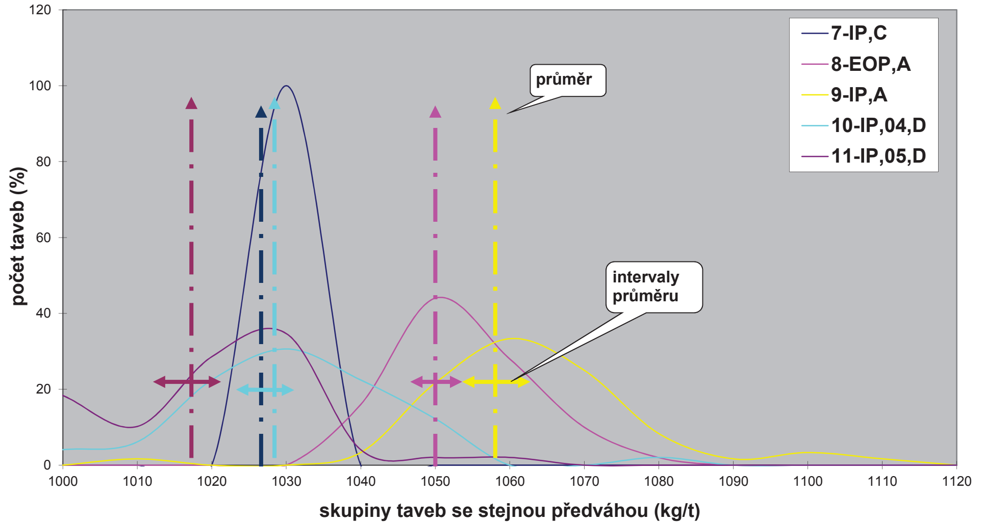
obr.5c: Relativní četnosti předváhy u výrobních způsobů "LKG"
