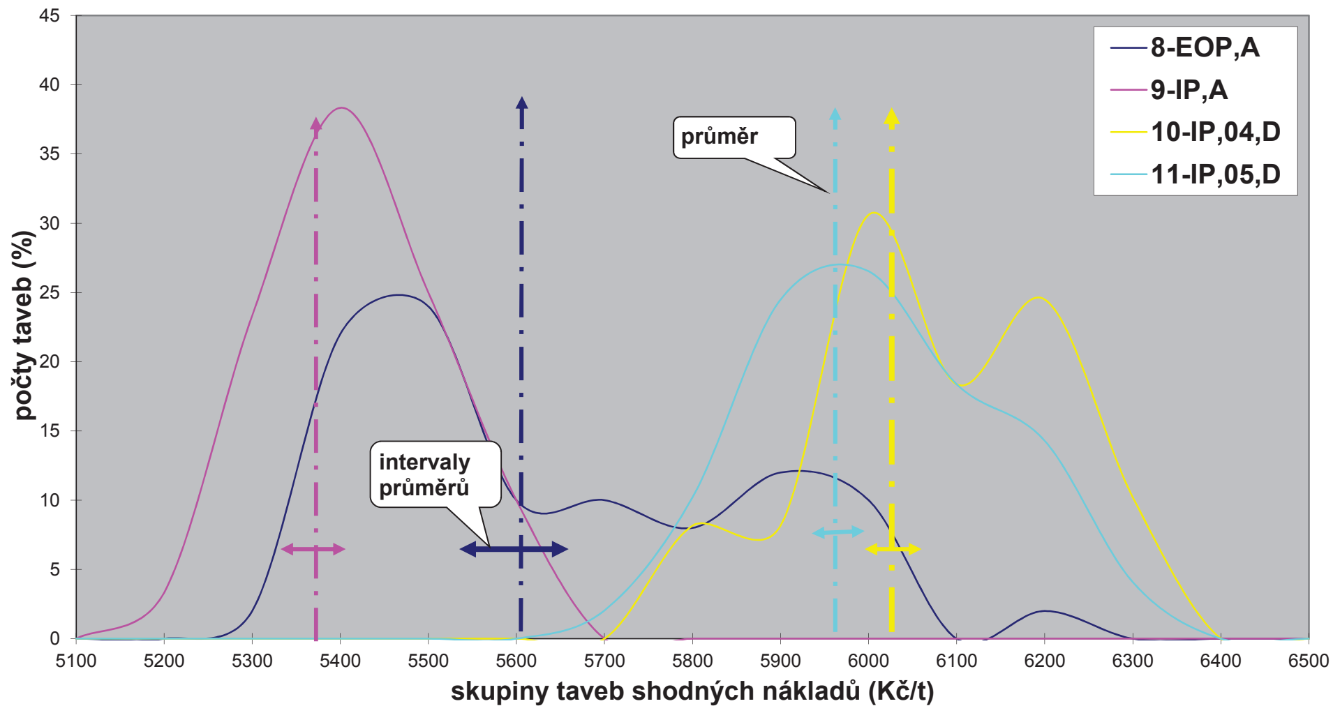
Obr.2c: Relativní četnosti nákladů na vsázku a přísady u výrobních způsobů "LKG"
