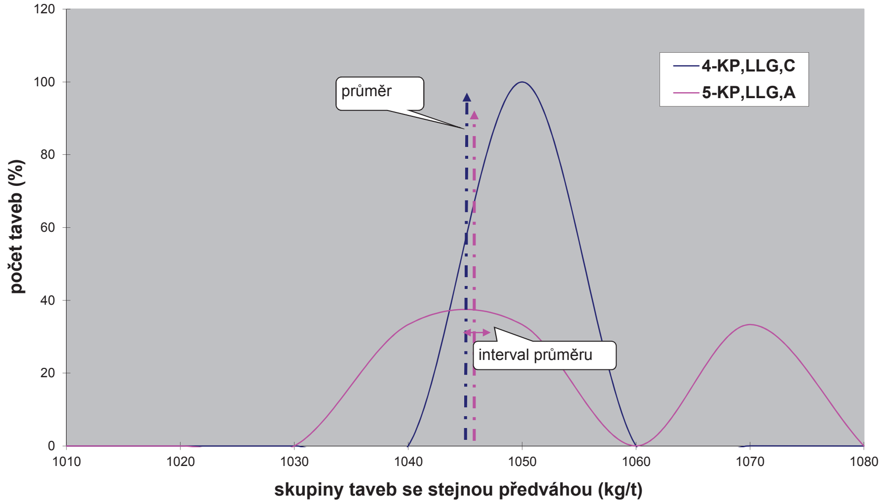
Obr.5b: Relativní četnosti předváhy u výrobních způsobů "LLG"
