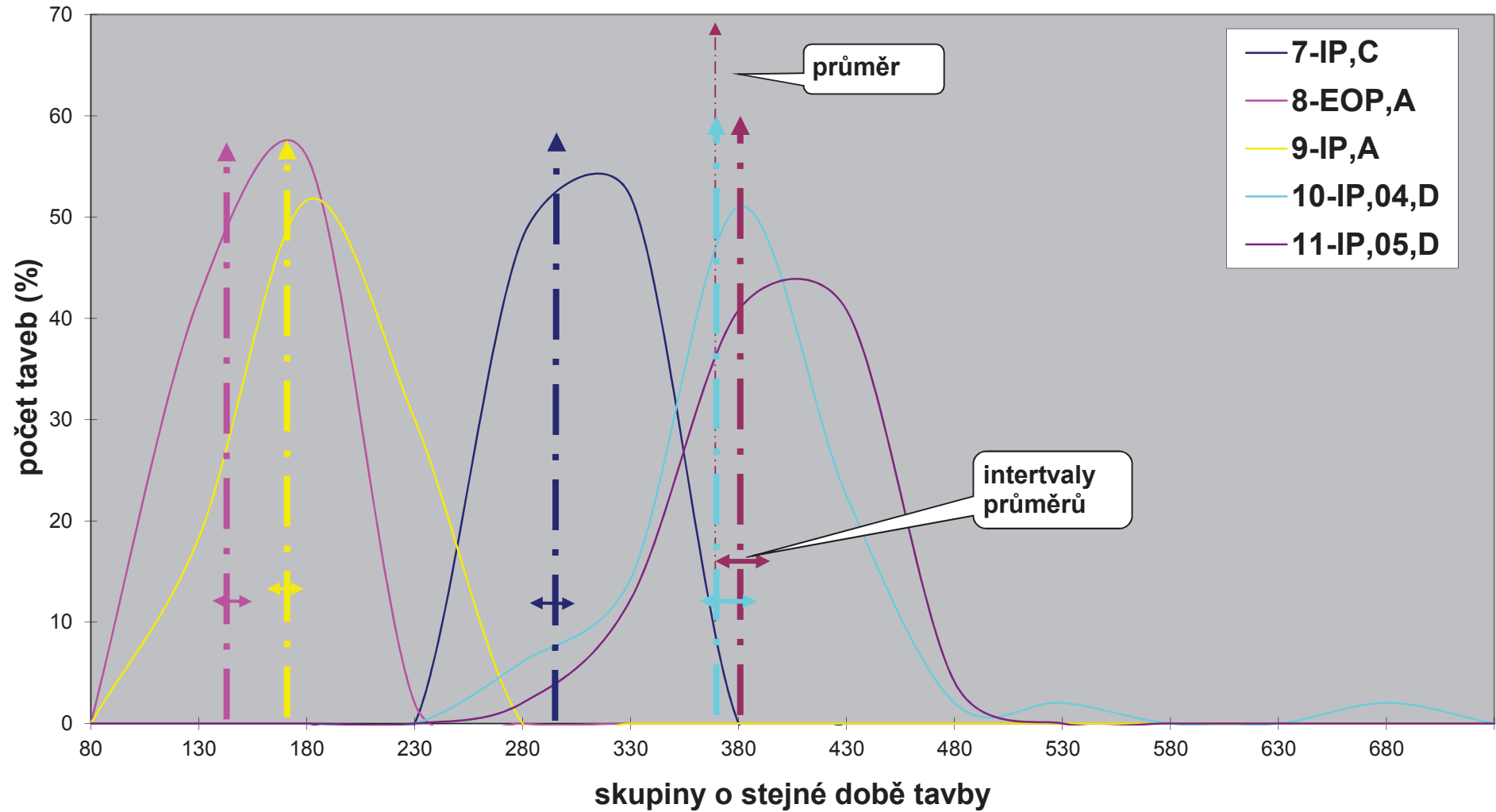
Obr.6c:Relativní četnosti dob tavby u výrobních způsobů "LKG"
